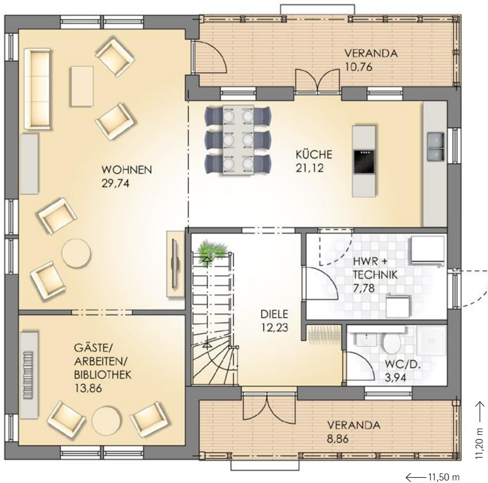
Erdgeschoss [Maßstab: ALA 1]
