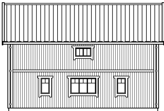
Seitenansicht rechts
