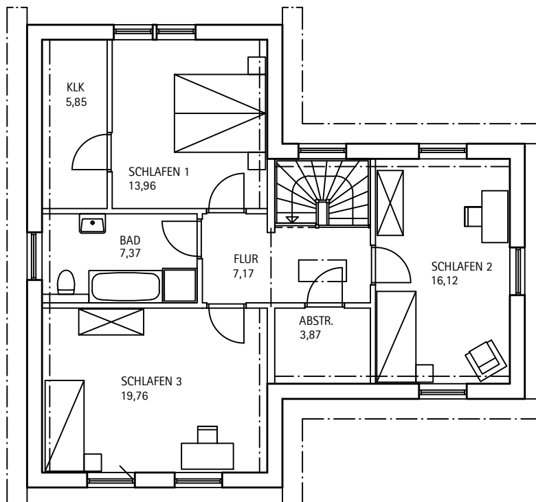
Obergeschoss
