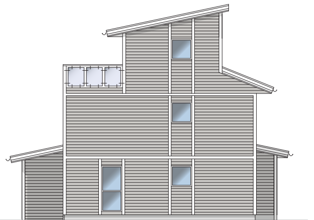
Seitenansicht links
