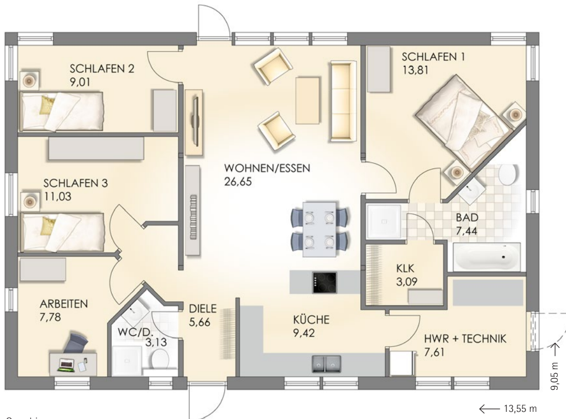
Grundriss [Maßstab: ALA 1]
