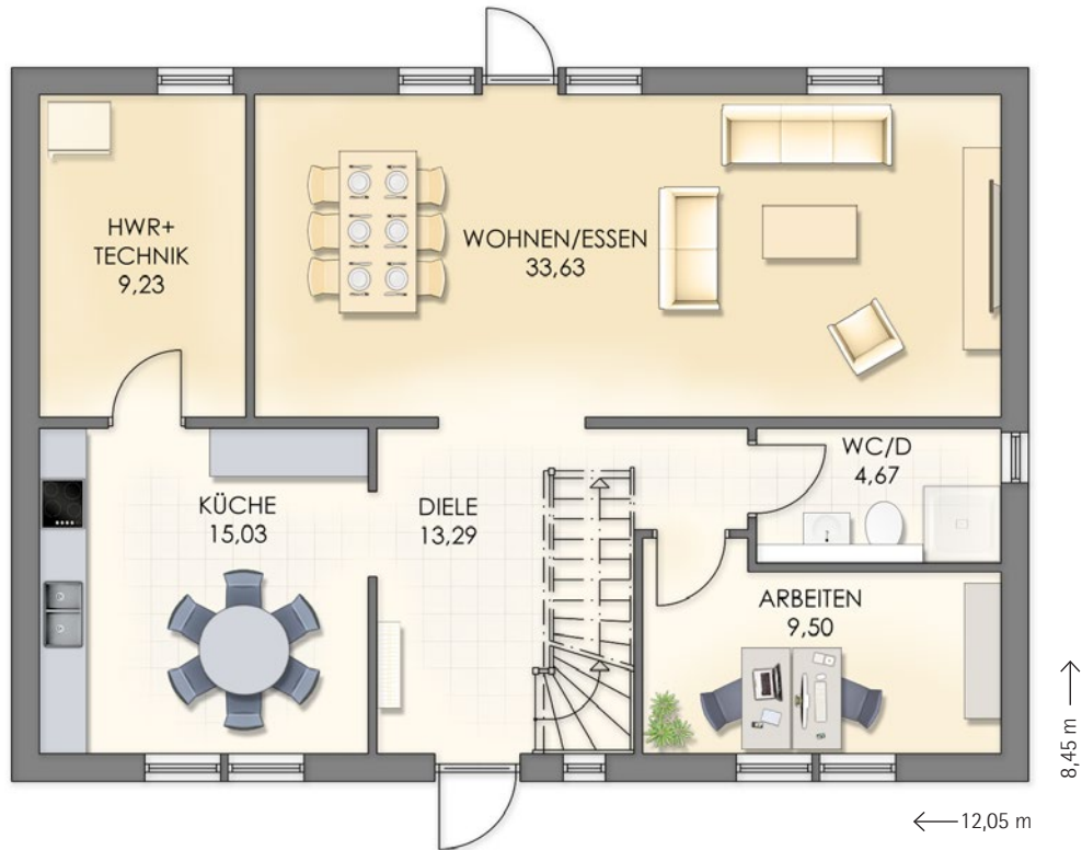
Erdgeschoss [Maßstab: ALA 1]
