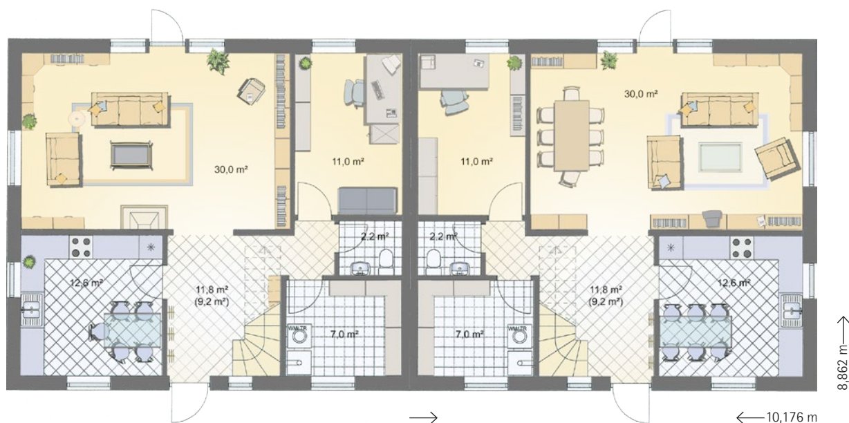
Erdgeschoss [Maßstab: ALA 2]
